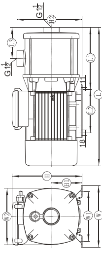
MTS-8 尺寸圖
